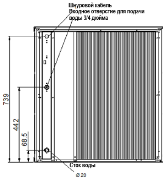
Воздушное охлаждение
