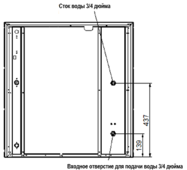
Водное охлаждение
