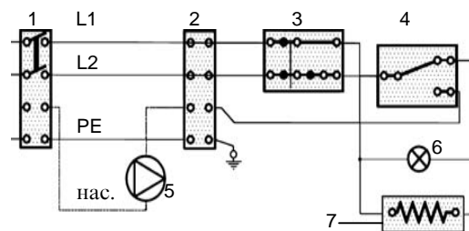
Рис. 3 Электросхема
