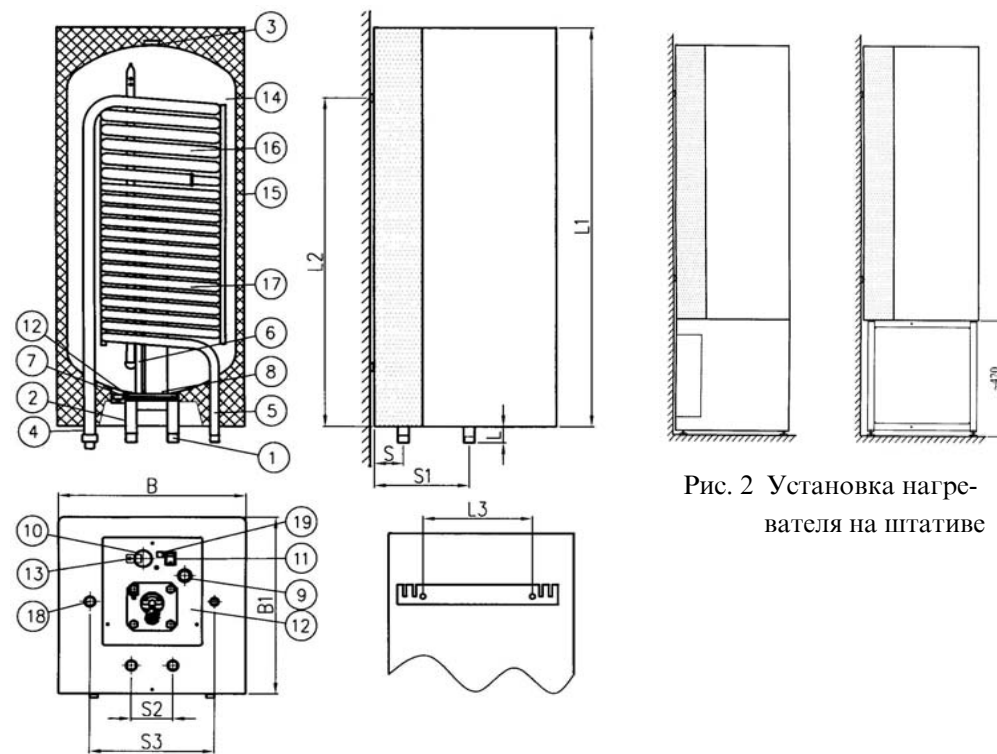
Рис. 1 Конструкция нагревателя
